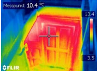
IR-Aufnahme Treppenabgang
